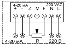
Токовый датчик ПТ-2*
