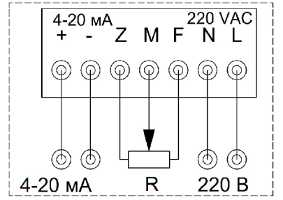
Токовый датчик ПТ-2
