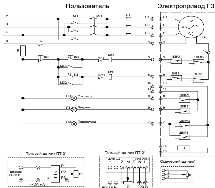
Рис.4 Электрическая схема управления
