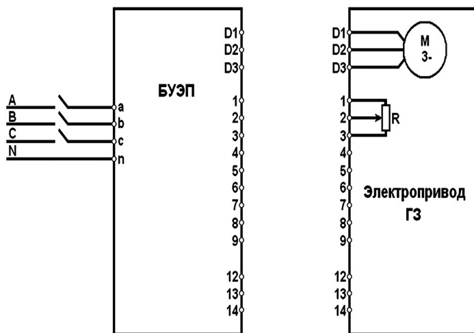
Рис.5 Блок-схема подключения БУЭП к электроприводу (для электросхемы на рис.4)
