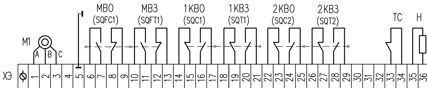
Диаграмма работы муфтовых концевых и путевых выключателей
